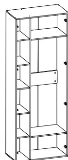
Корпус 32 800 x 414 x 1950
