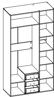
Корпус 3 1200 x 540 x 2272
