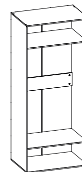
Оскар 2 800 x 540 x 2272
