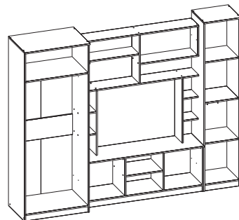
2700 x 544 x 2100 размер ниши под ТВ 1040 x 800
