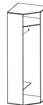
Корпус 25 726 x 726 x 2272
