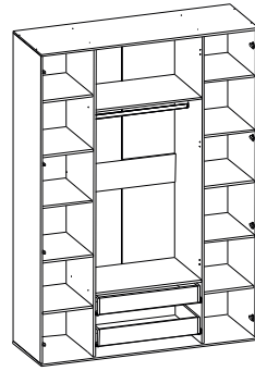
Корпус 4 1600 x 540 x 2272
