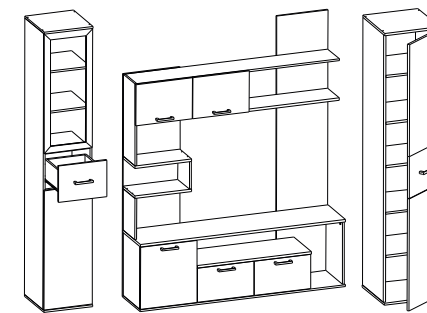
NEXT ГОСТИНАЯ 2 2554 x 414 x 2272
