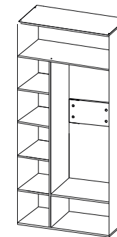
Оскар 22 800 x 414 x 2272
