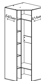
Корпус 25-5 852 x 726 x 2272
