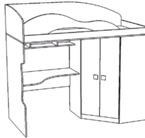
Кровать 2-этаж + шкаф 2032 x 1870 x 852
