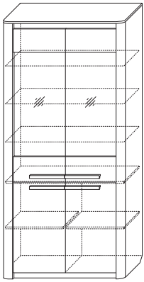
1 ГТ.0118.301 Шкаф со стеклом 1050 x 2200 (ВхШхГ): 2200 x 1050 x 480
