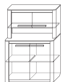
11 ГТ.0118.311 Шкаф с нишей 1050 x 1550 (ВхШхГ): 1550 x 1050 x 480
