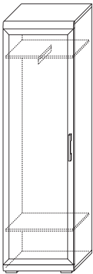
6 ГТ.016.308 ↔ Шкаф для одежды 600 x 414 3 (ВхШхГ): 2126 x 600 x 414
