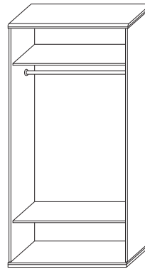
■ СП.014.402 Шкаф 2-х дверный (корпус) (ВхШхГ): 2227 x 968 x 574
