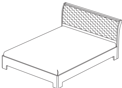
■ СП.0410.406 / 407 / 401 / 402 / 403 Кровать-3 с ортопедическим основанием 900 / 1200 / 1400 / 1600 / 1800 (ВхШхГ): 930 x 955 / 1255 / 1455 / 1655 / 1855 x 2245
