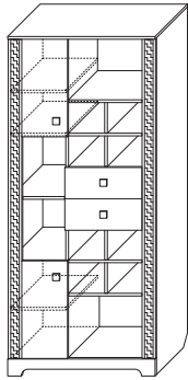
2 ГТ.0119.302 Шкаф открытый 870 (2 двери, 2 ящика) (ВхШхГ): 2000 x 870 x 450
