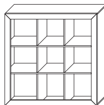
22 ГТ.0717.309 Полка 1200 x 1200 (ВхШхГ): 1200 x 1200 x 350
