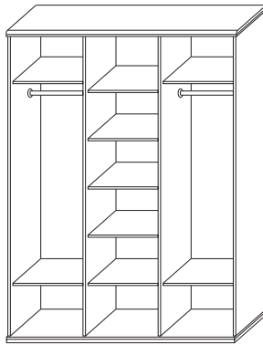
■ СП.014.403 Шкаф 3-х дверный (корпус) (ВхШхГ): 2227 x 1450 x 574
