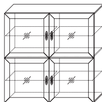
21 ГТ.0717.308 4☀ Полка 1200 x 1200 (4 стеклодвери) (ВхШхГ): 1200 x 1200 x 350
