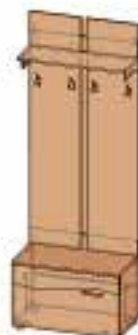
Вешалка с тумбой Д 750 x В 2110 x Г 403 мм
